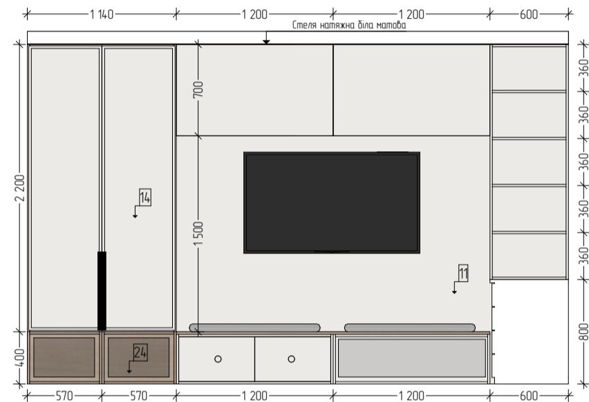
22 Розгортка 1:40
