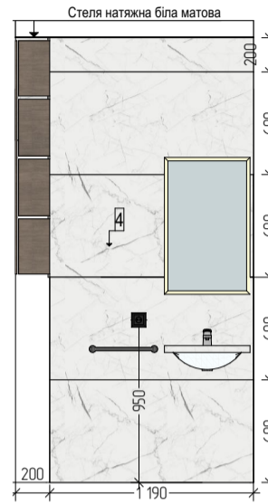
7 Розгортка 1:40
