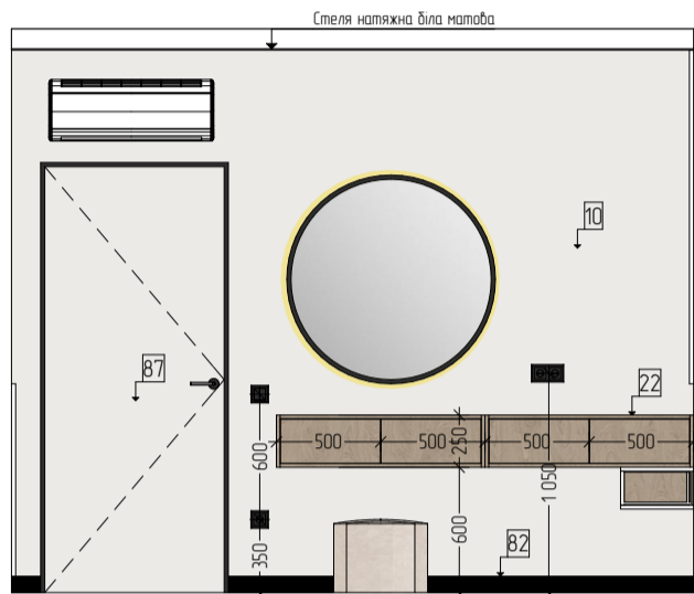
25 Розгортка 1:40
