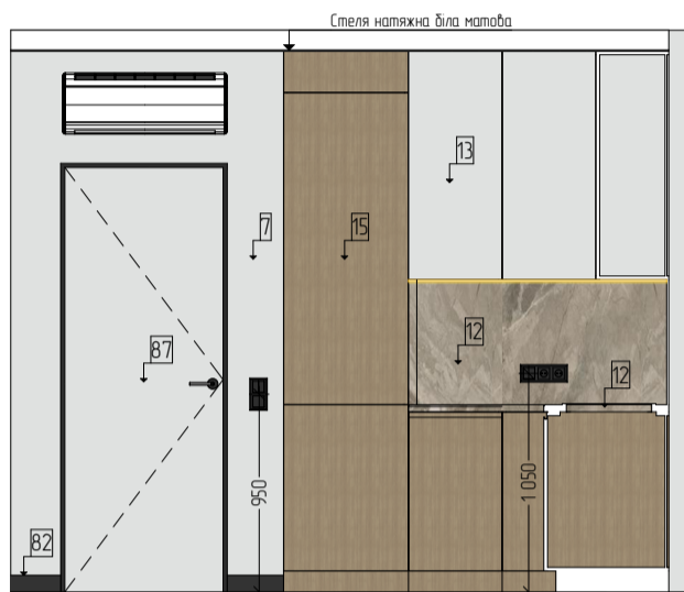
13 Розгортка 1:40
