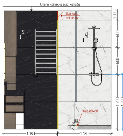
11 Розгортка 1:40
