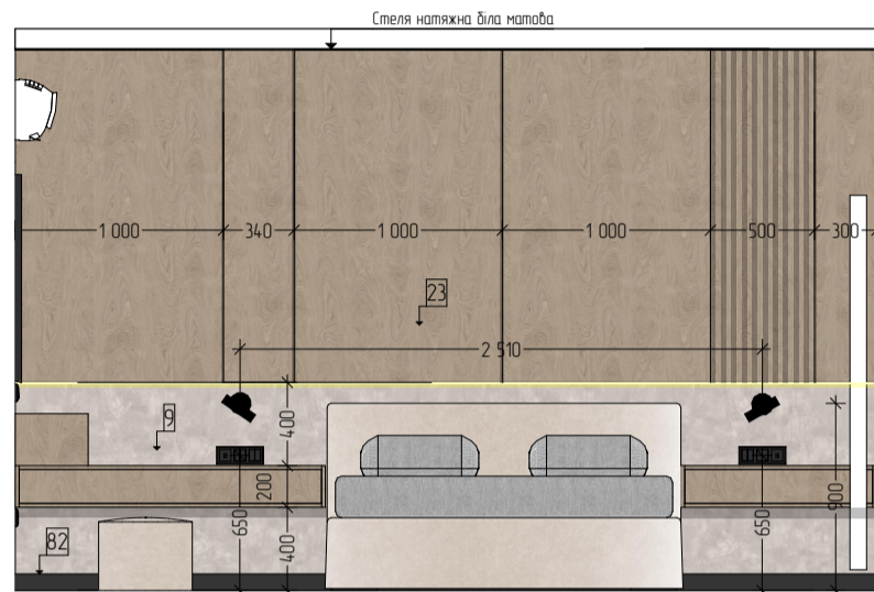
26 Розгортка 1:40
