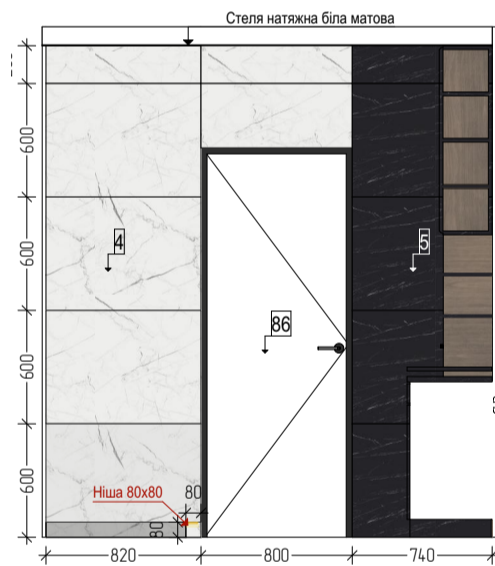
9 Розгортка 1:40
