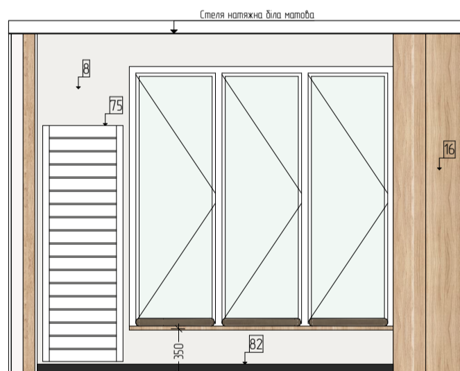
17 Розгортка 1:40
