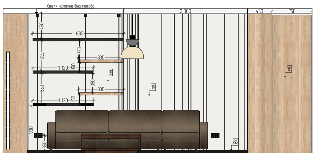
18 Розгортка 1:40
