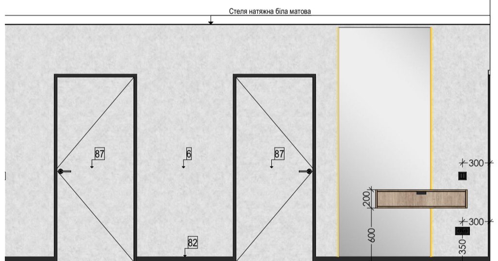
4 Розгортка 1:40
