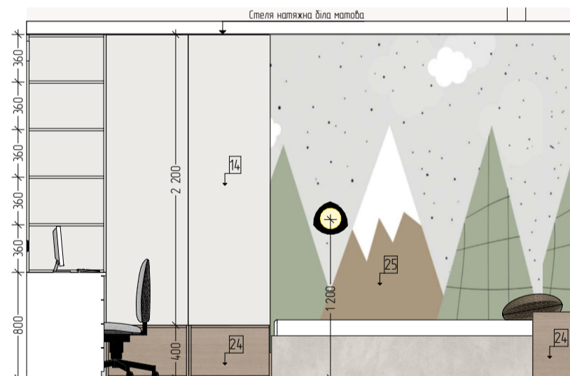
24 Розгортка 1:40
