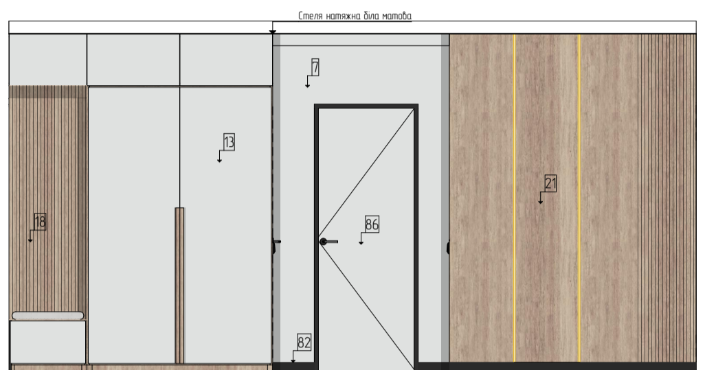
2 Розгортка 1:40
