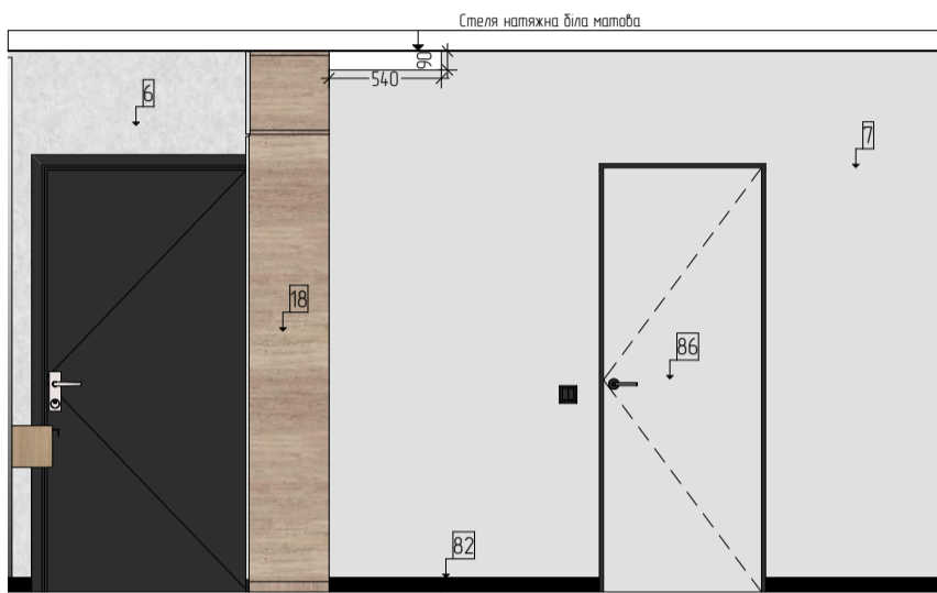
1 Розгортка 1:40
