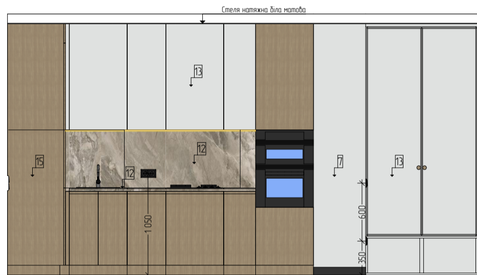
14 Розгортка 1:40
