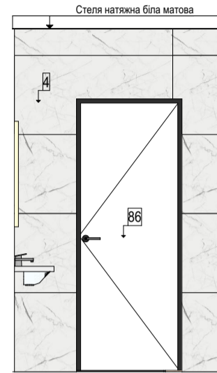
8 Розгортка 1:40
