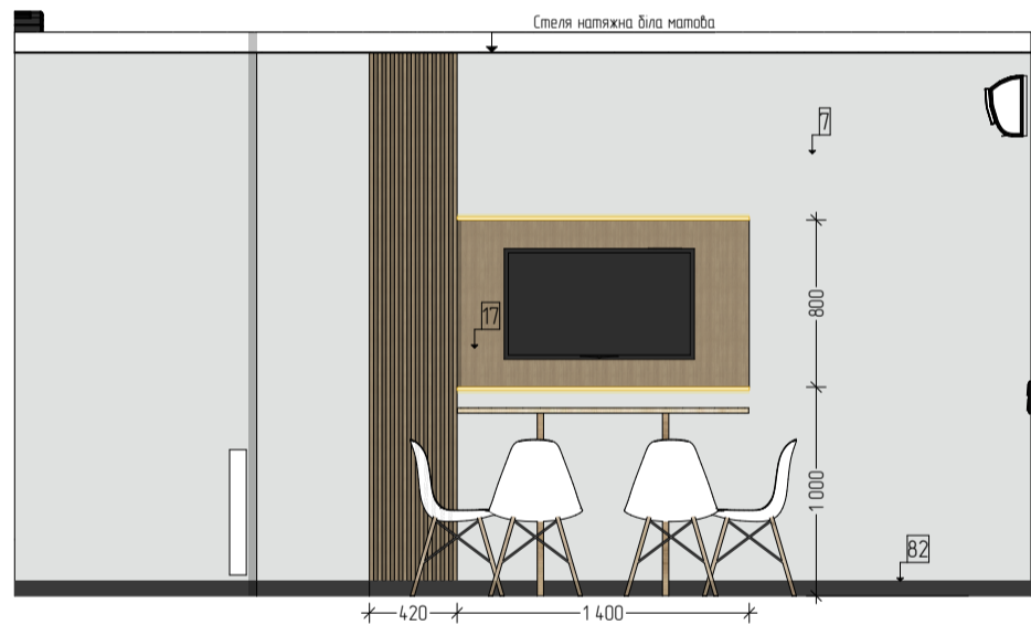
16 Розгортка 1:40
