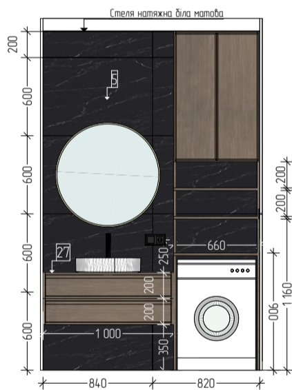
10 Розгортка 1:40
