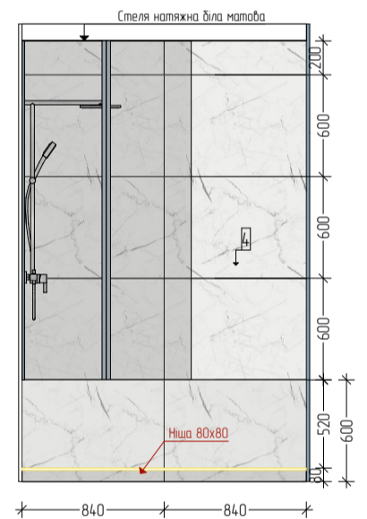
12 Розгортка 1:40
