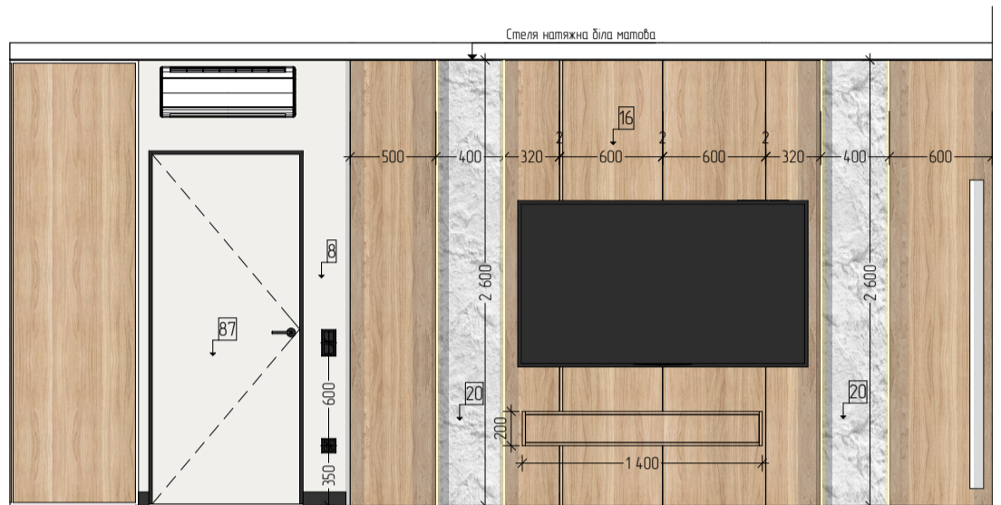
18 Розгортка 1:40
