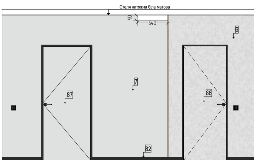
3 Розгортка 1:40
