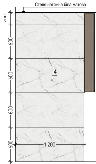
5 Розгортка 1:40
